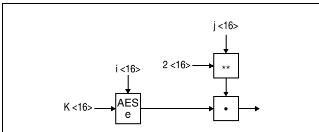
Figure 7-286. Compute XTS Parameter Using AES 128
