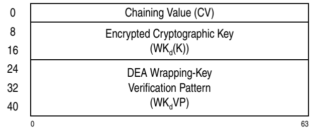
Figure 7-88. Parameter Block for KMF-TDEA-128
