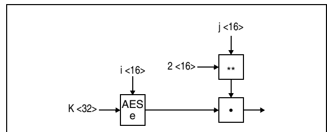
Figure 7-289. Compute XTS Parameter Using AES 256
